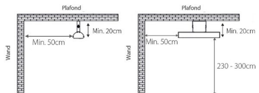
plafondmontage
