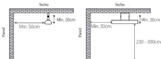
techo montado
