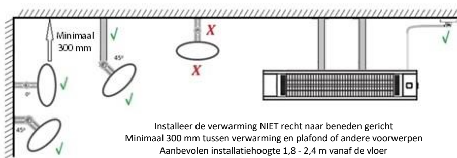
Diagram 2: Correcte positie wand / plafond
