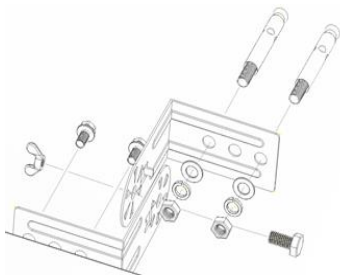
Diagramm 3: Halterungsmontage
