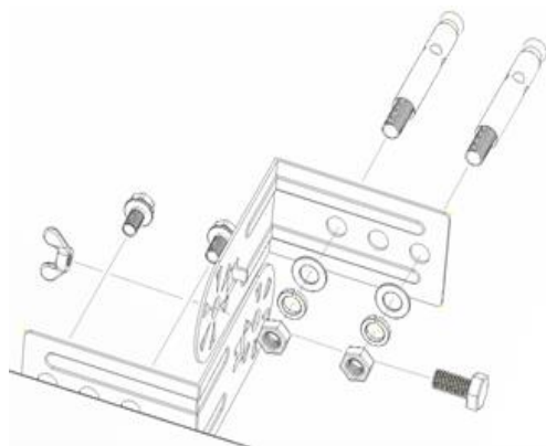
Diagrama 3: Montaje del soporte
